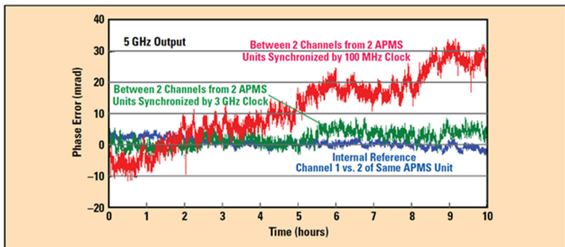
Figure 1: Phase stability measured over 10 hours. 在 10 小时内测得的相稳定性
